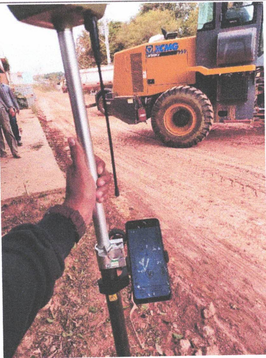
MARCAÇÃO TOPOGRAFICA
