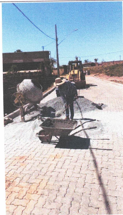
EXECUÇÃO DE CONCRETO PARA SARJETA
